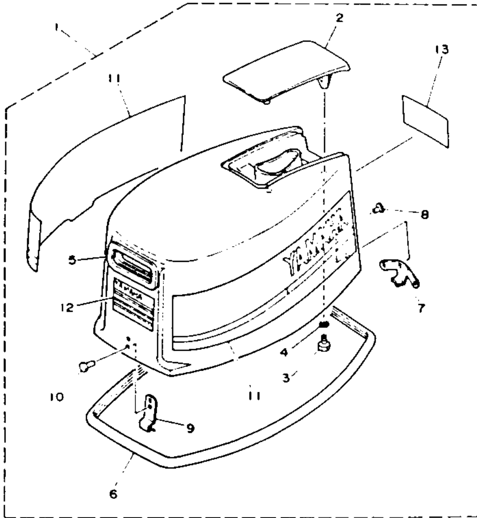
C25ELRP 1991 / TOP COWLING
