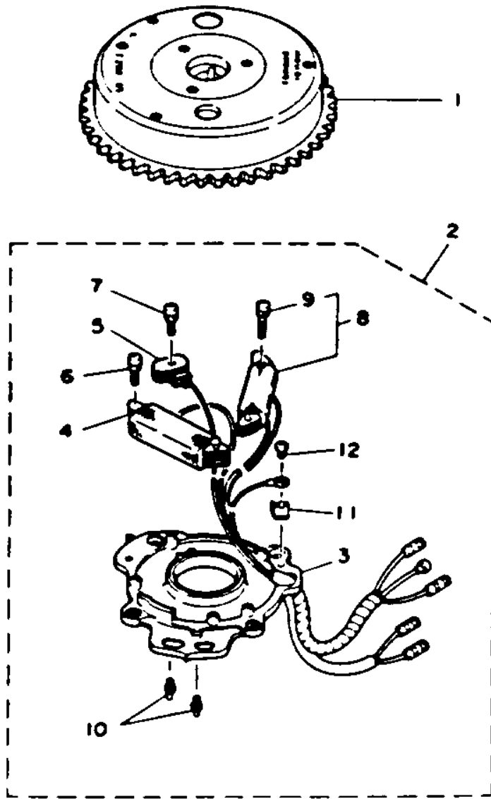
15ESHR 1993 / CDI MAGNETO (9.9E 15E)
