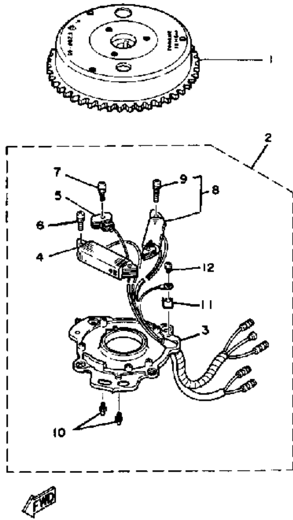
15ELJ 1986 / CDI MAGNETO (9.9EH 15EH)
