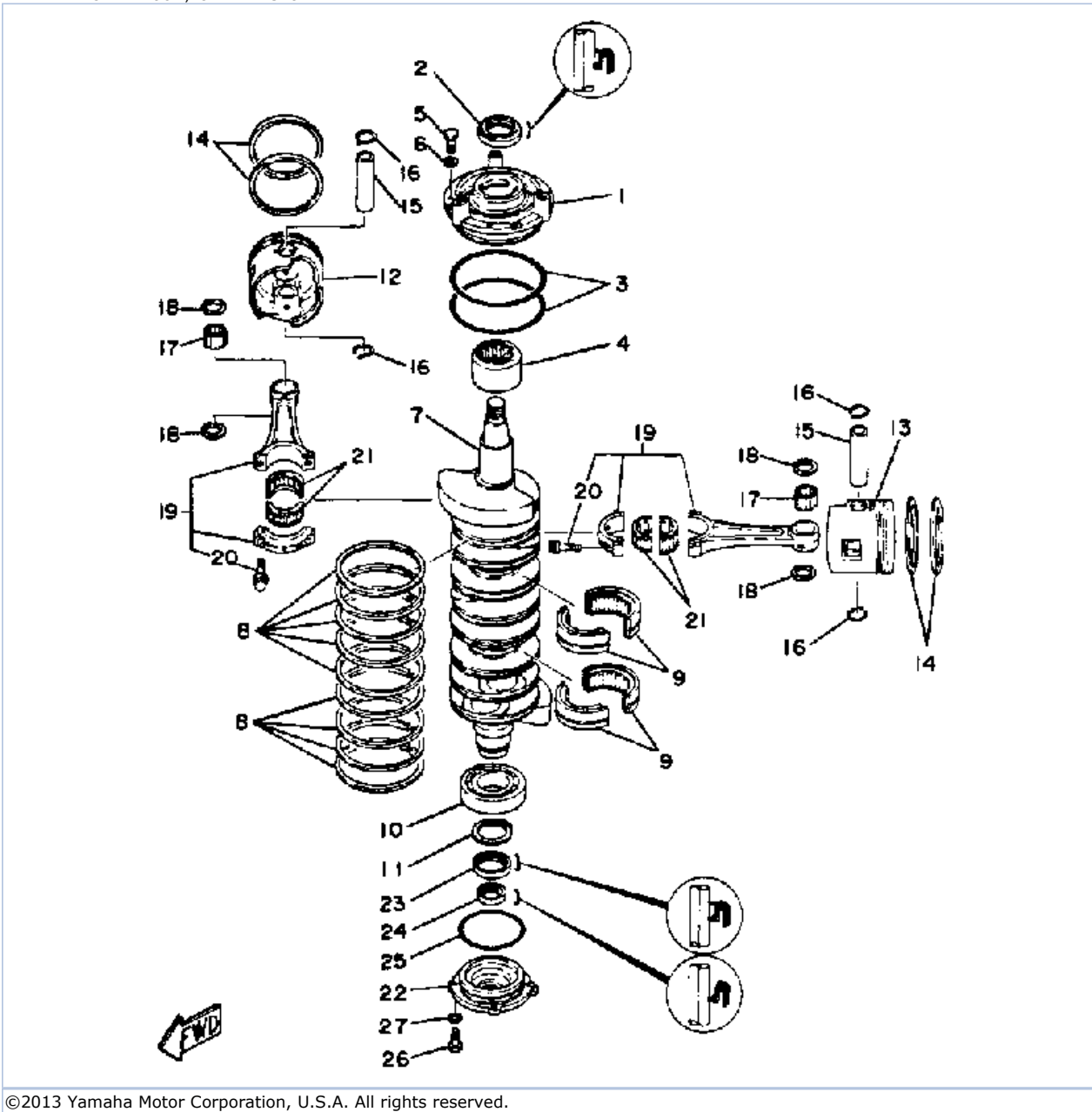
175ETLN 1984 / CRANK PISTON
