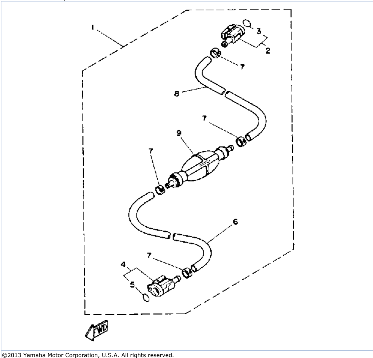
150ETXH 1987 / FUEL SYSTEM 2
