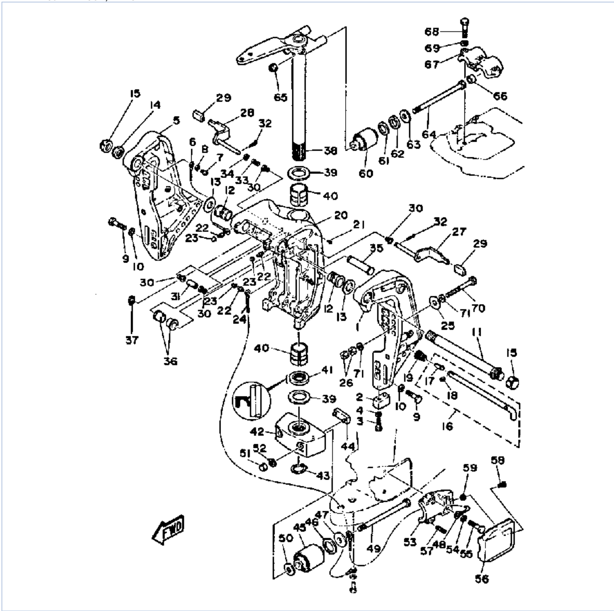
150ETXH 1987 / BRACKET
