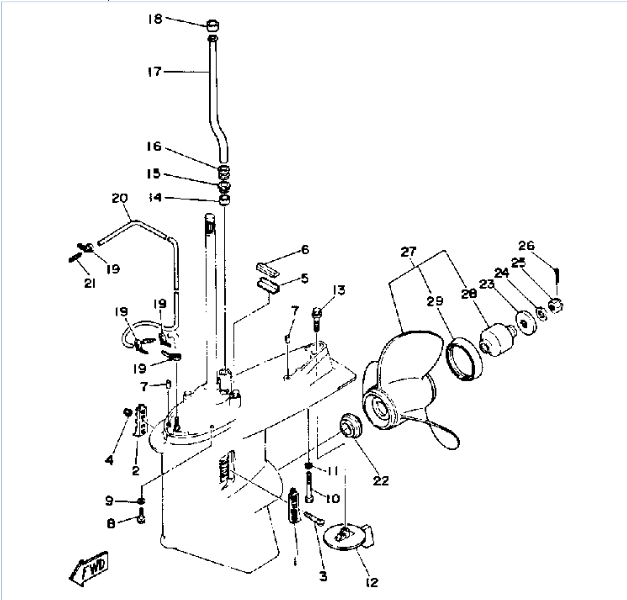
150ETXH 1987 / LOWER DRIVE 2
